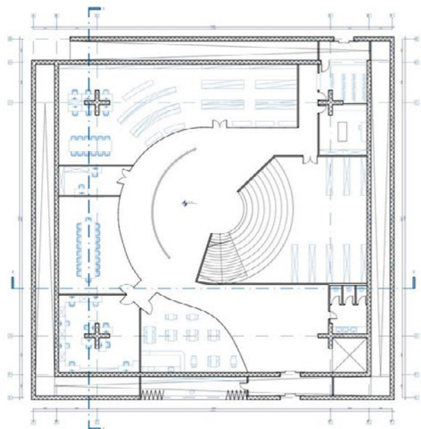
osnova prizemlja
