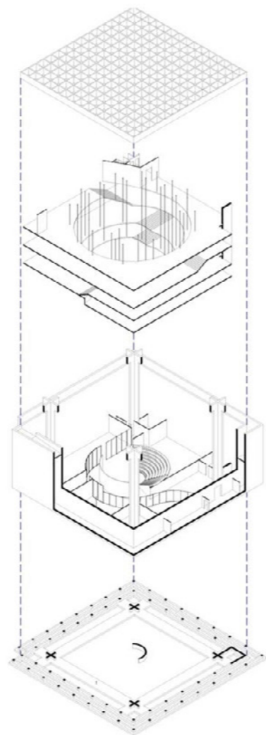
eksplozirana izometrija
