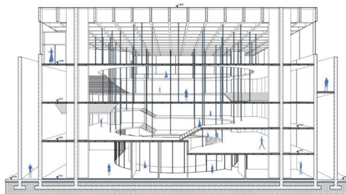
presek 1-1
